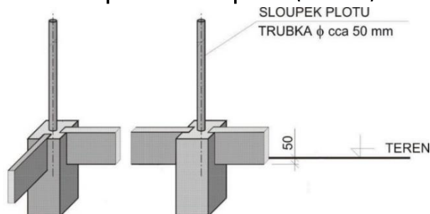
Patka plotová + Deska plotová (standard)
