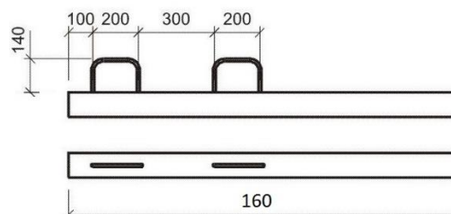
Sloupek pro elektrický ohradník
