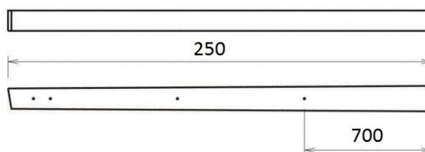
Sloupek ohradníkový Typ 160 (OKA)
